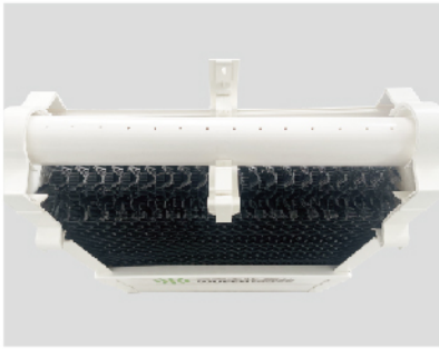
滴淋管 \phi 63
