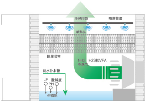
纵向通风除臭模式示意图
