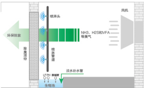
水平通风除臭模式示意图
