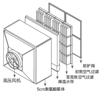
空气过滤模块典型结构型式示意图
