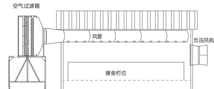
季节性空气过滤模式典型结构类型示意图
